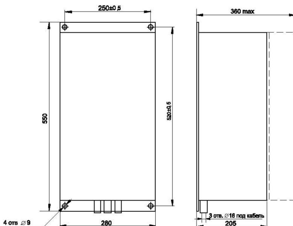
Рис. 42. Габаритные и установочные размеры стабилизатора напряжения ИСН-М
