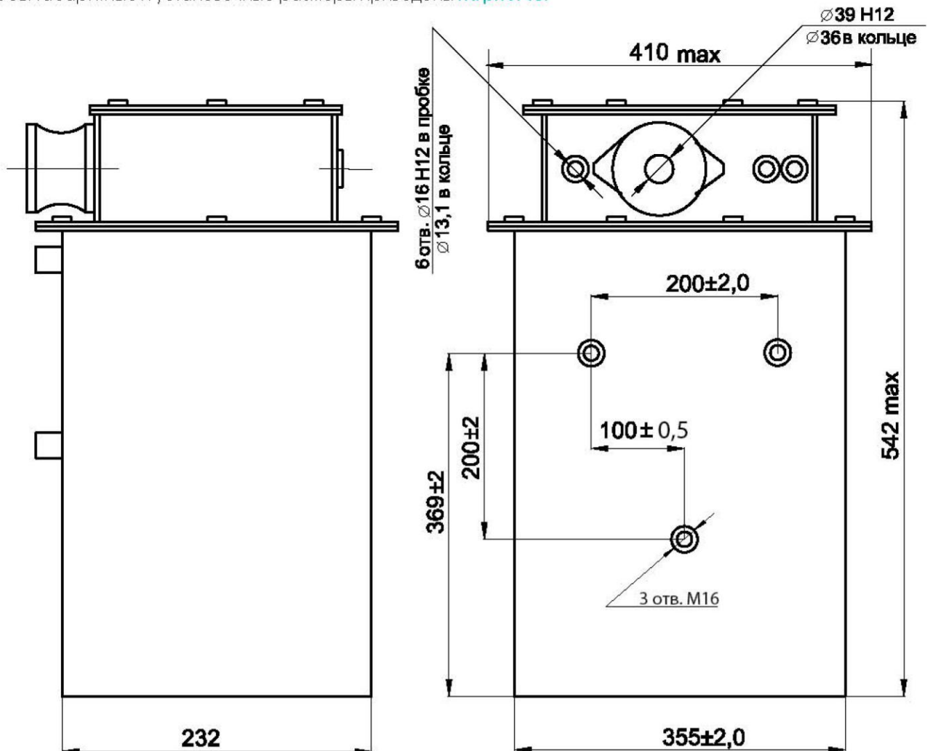
Рис. 48. Габаритные и установочные размеры блоков диодов БД-2М
