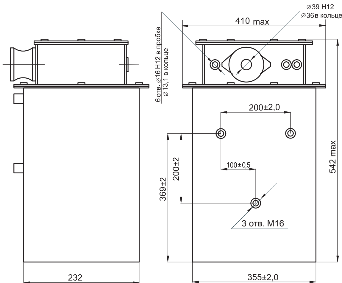
Рис. 50. Габаритные и установочные размеры блоков диодов БД-2М
